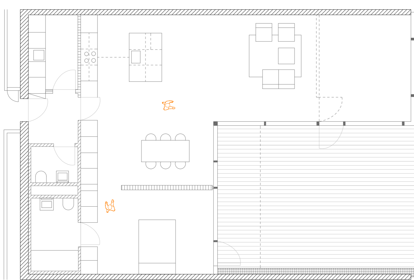
Vivienda tipo I
